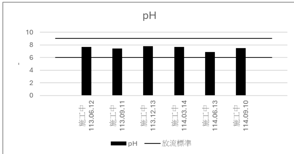
圖 2.4-2 放流水質監測結果(pH)
