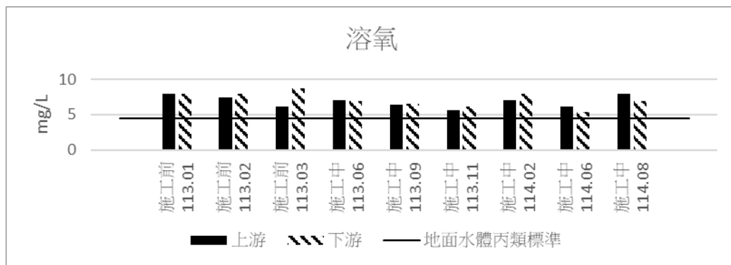
圖 2.3-5 河川水質監測結果(溶氧)
