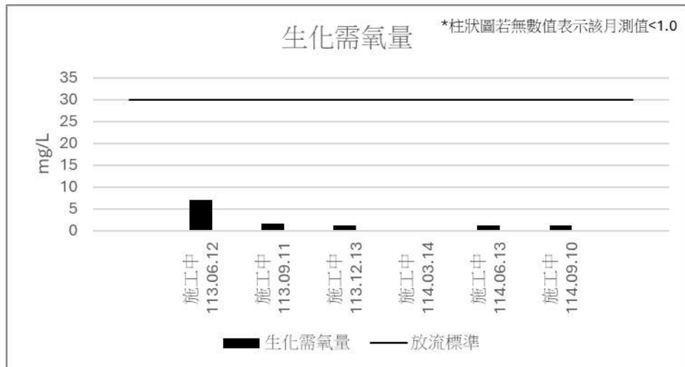
圖 2.4-4 放流水質監測結果(生化需氧量)
