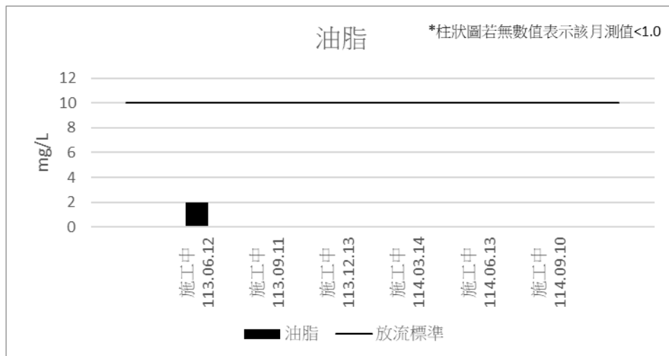
圖 2.4-5 放流水質監測結果(油脂)
