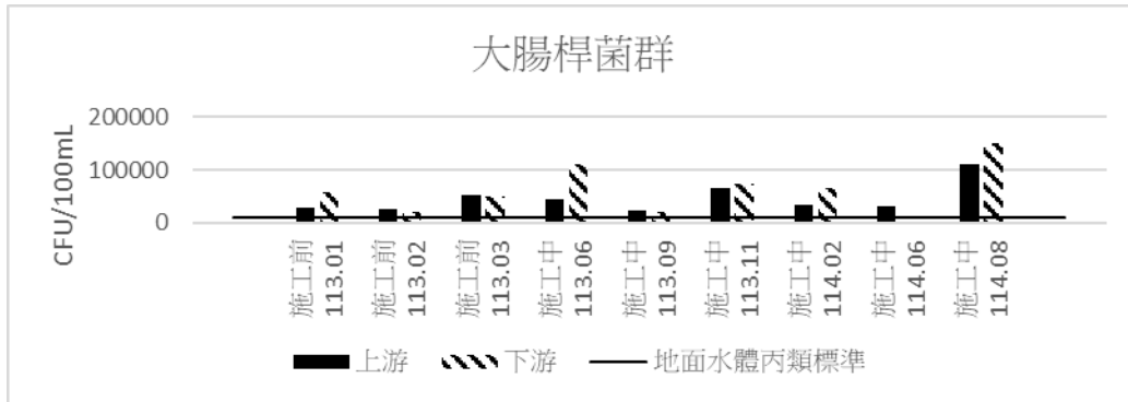
圖 2.3-1 河川水質監測結果(大腸桿菌群)
