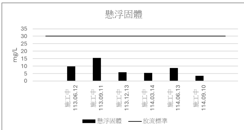
圖 2.4-3 放流水質監測結果(懸浮固體)
