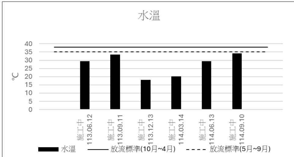
圖 2.4-1 放流水質監測結果(水溫)
