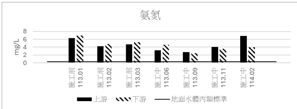
圖 2.3-4 河川水質監測結果(氨氮)
