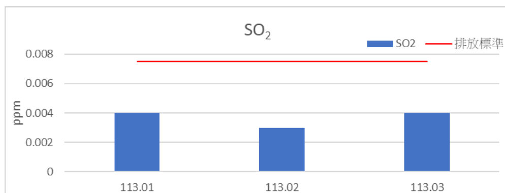
圖 3.1-1 空氣品質監測結果(SO 2 )
