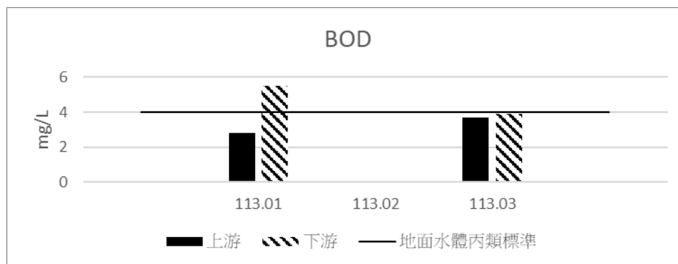
圖 3.3-6 河川水質監測結果(BOD)
