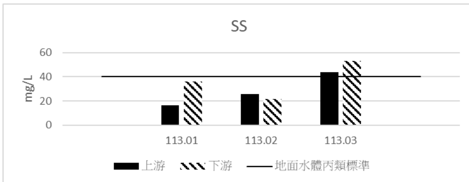
圖 3.3-2 河川水質監測結果(SS)
