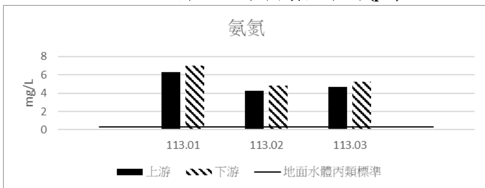
圖 3.3-4 河川水質監測結果(氨氮)
