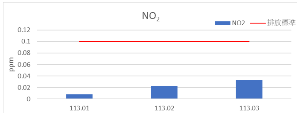
圖 3.1-2 空氣品質監測結果(NO 2 )
