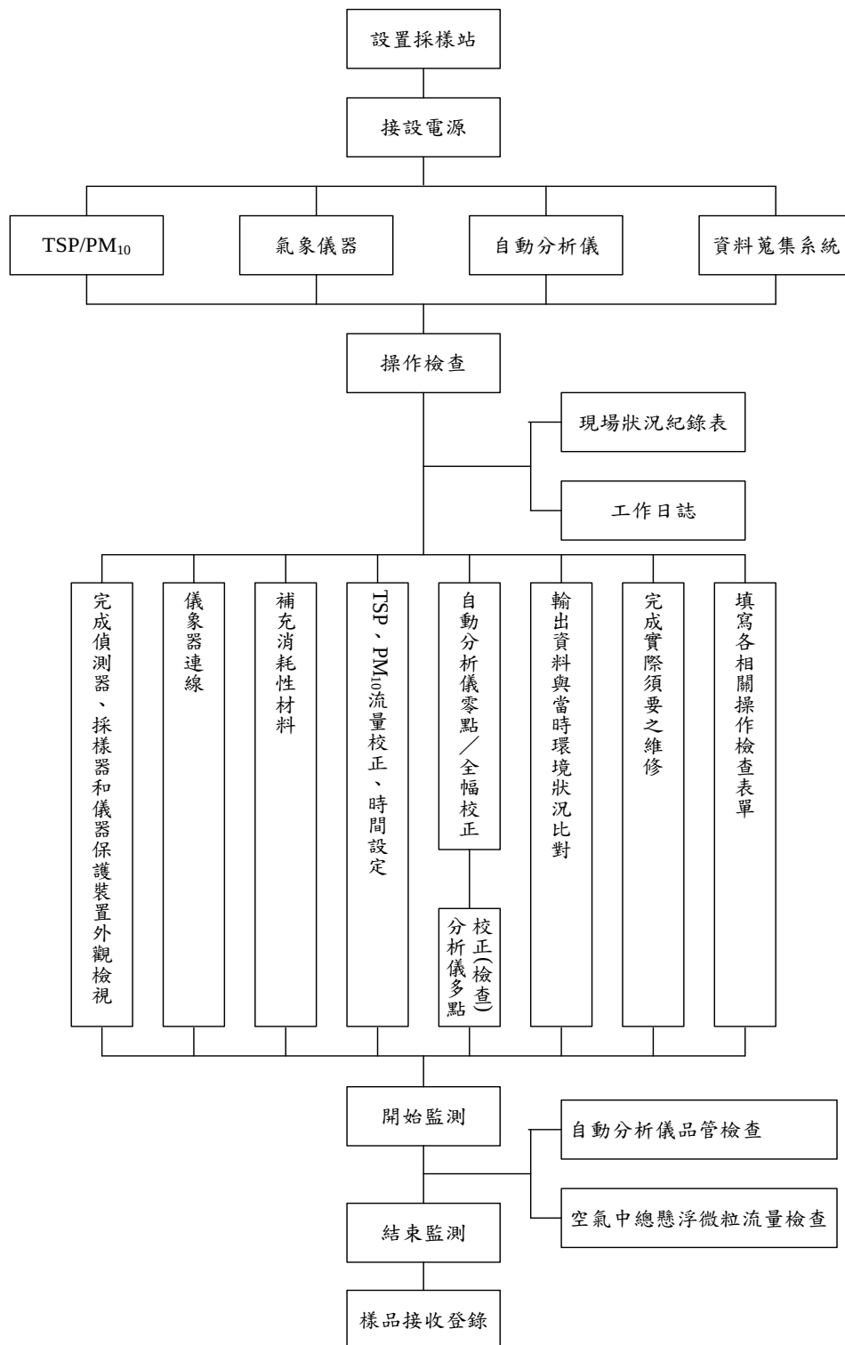
圖 2.8-2 空氣採樣作業流程圖
