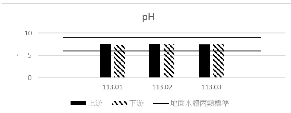
圖 3.3-3 河川水質監測結果(pH)
