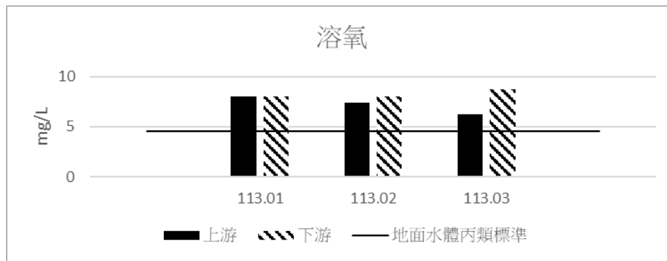
圖 3.3-5 河川水質監測結果(溶氧)
