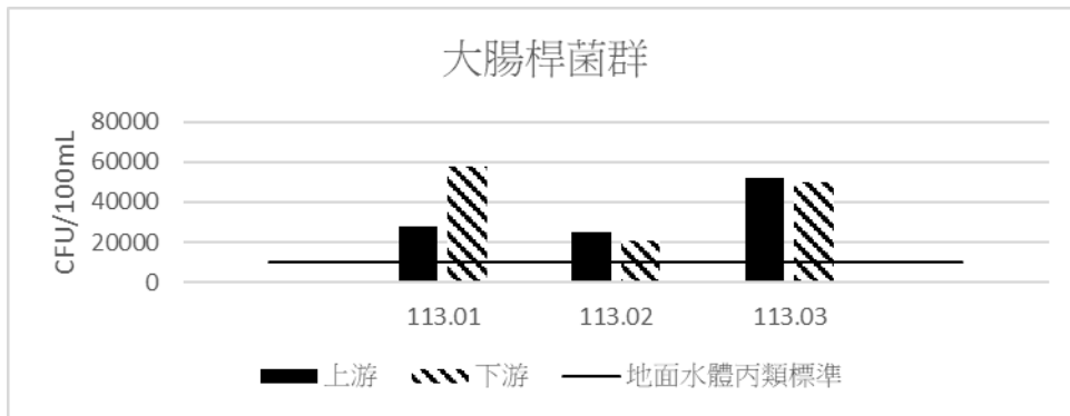
圖 3.3-1 河川水質監測結果(大腸桿菌群)
